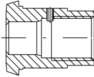
COUPLINGS DIN11887-STANDARD :
